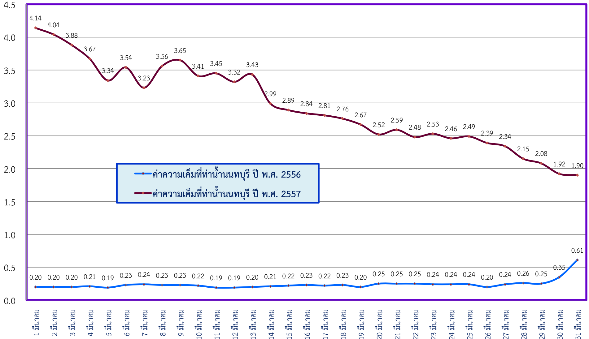
กราฟแสดงการเปรียบเทียบค่าความเค็มในแม่น้ำเจ้าพระยา ที่จุดตรวจวัดทำนายนนทบุรี เดือนมีนาคม 2556 กับ 2557
